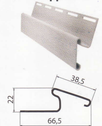
Переходник вертикального сайдинга
