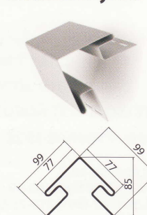
Внешний угол
