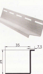
Сливная планка
