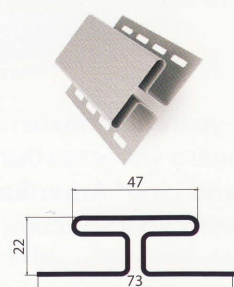
Н-профиль соединительный
