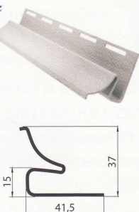
Молдинг
