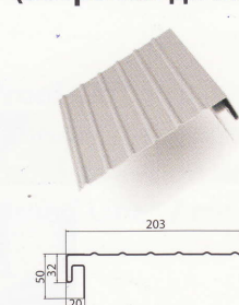
Ветровая доска
