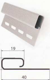
Финишная планка
