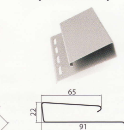
Ветровая доска
