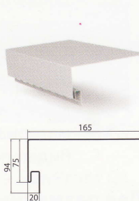
Приоконная планка
