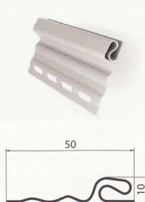
Стартовая планка
